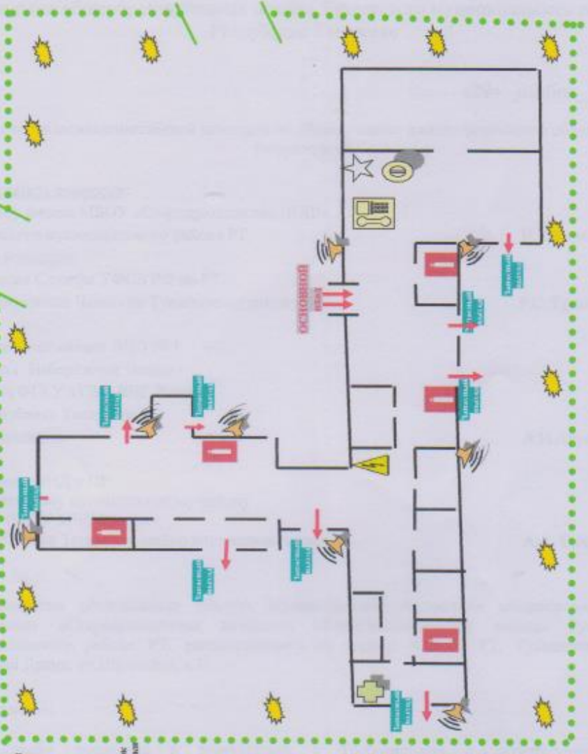
План (схема) охраны объекта (территории) с указанием контрольно-пропускных пунктов, постов охраны, инженерно-технических средств охраны МБОУ «Стародомовская НОШ» Тукаевского района
